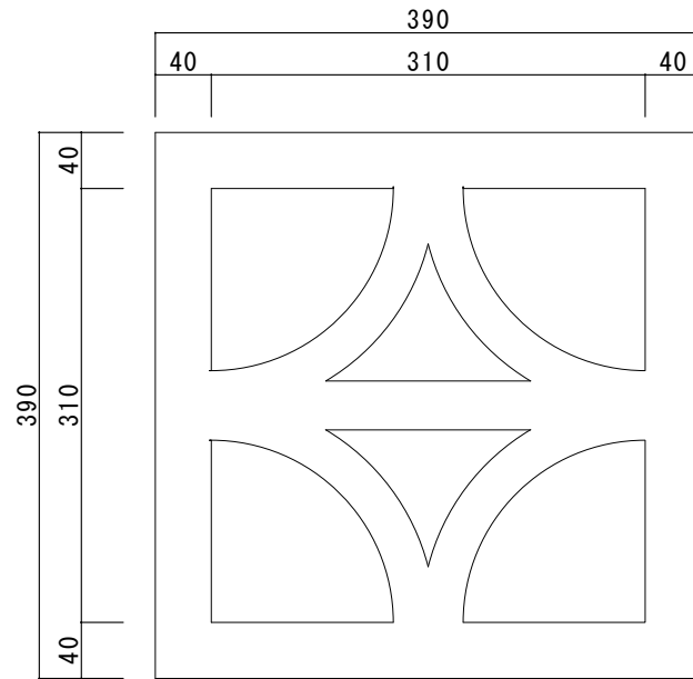
正面図
